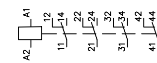
NOKKAKYTKIMET+RELEET
